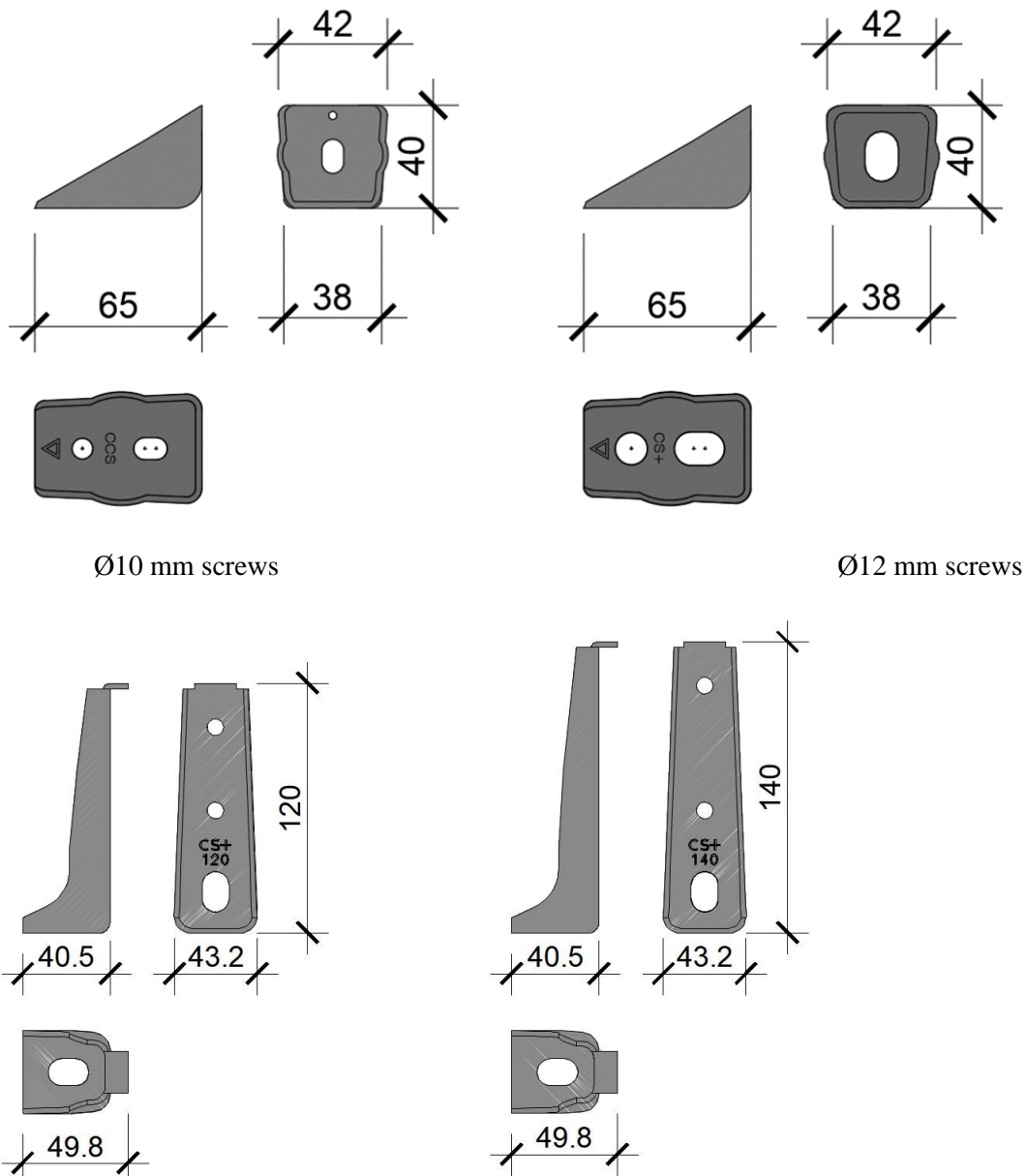
Figure 1.1.e LATERLITE CONNETTORE CENTROSTORICO LEGNO without screw
